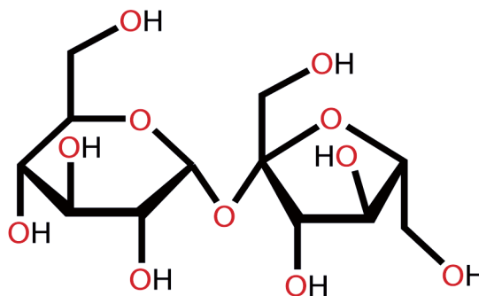
Esquema del enlace glucosídico en la sacarosa.
